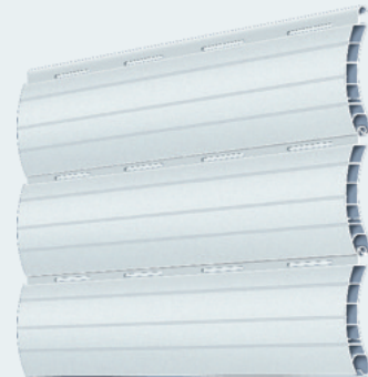
Rolluiklamellen Typ Z55 De Z55 met vierpuntsstabilisatie maakt breedtes tot 2,60 m mogelijk.
